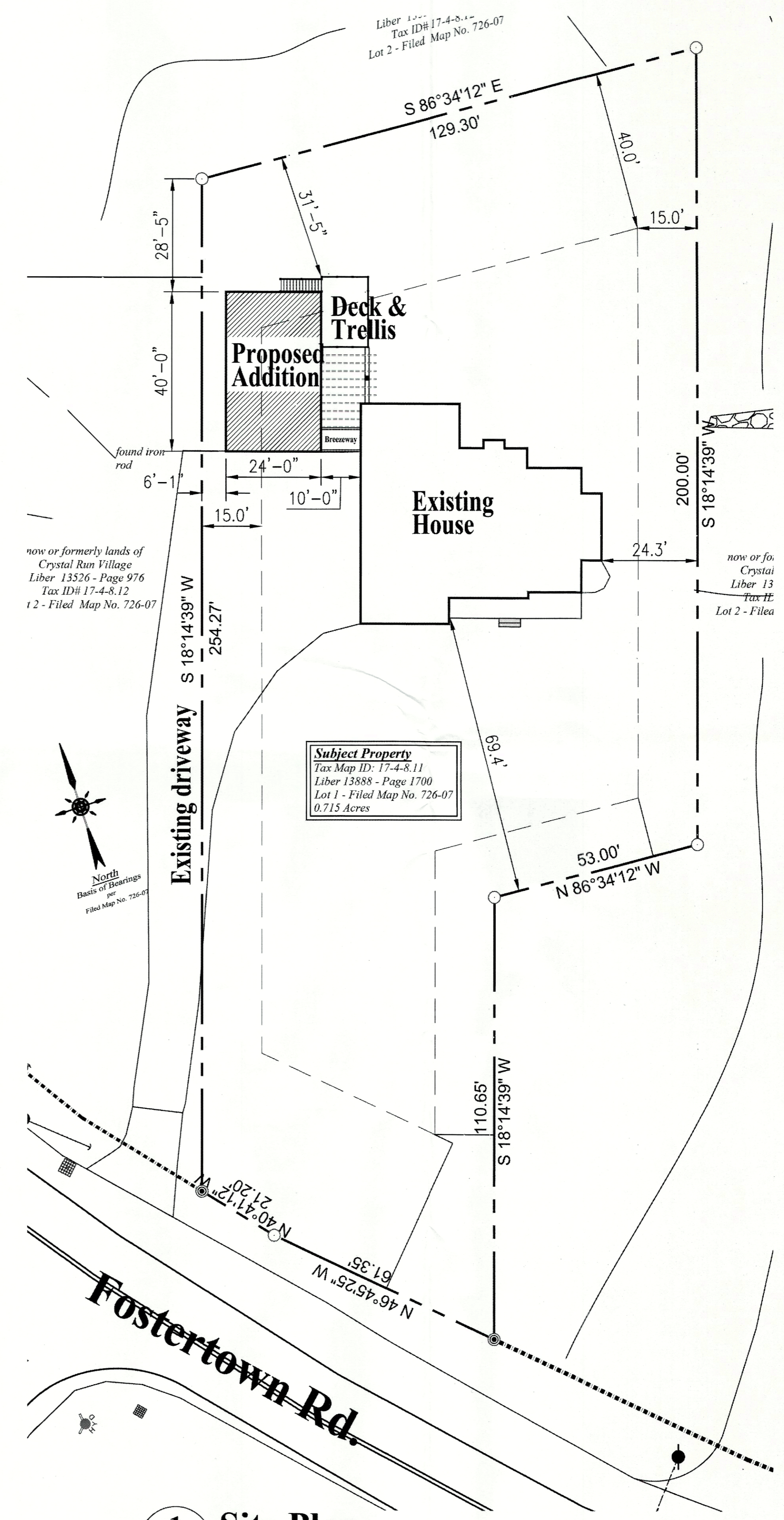
1 Site Plan A2 Scale: 1"=20'-0"
