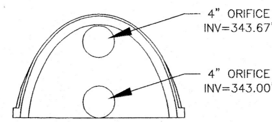
STORMTECH SC-310 CHAMBER OUTLET END SECTION N.T.S.
