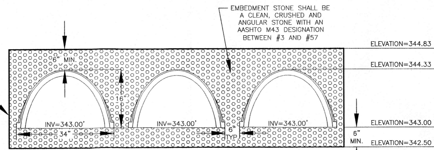
STORMTECH SC-310 CHAMBER OUTLET END SECTION N.T.S.
