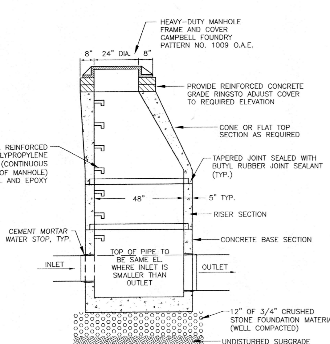
DRAINAGE MANHOLE DETAIL N.T.S.
