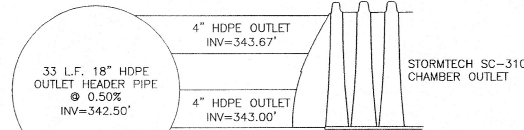
STORMTECH SC-310 CHAMBER OUTLET N.T.S.
