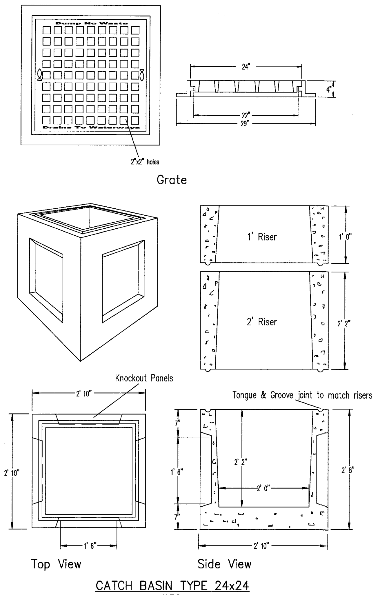
CATCH BASIN TYPE 24x24 N.T.S.
